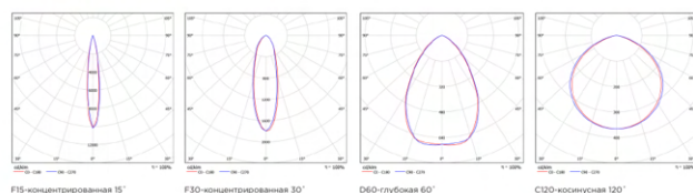
Тип кривой силы света
